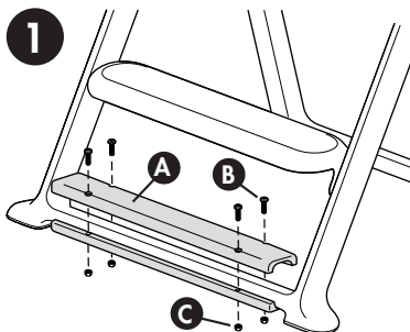
A Contrapesos (x2) Gewichte (x2)
